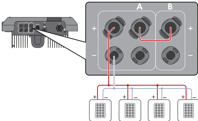
Figur 10: Översikt för anslutningen vid parallellkoppling av likströmsingångarna A och B
