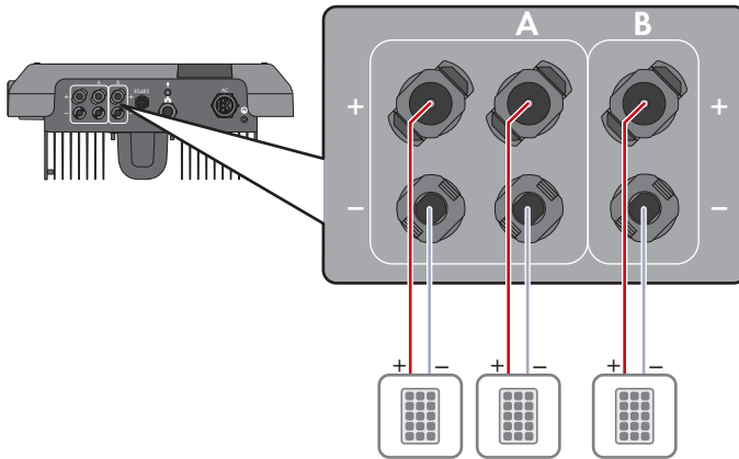
Figur 9: Översikt för anslutningen vid normal drift
