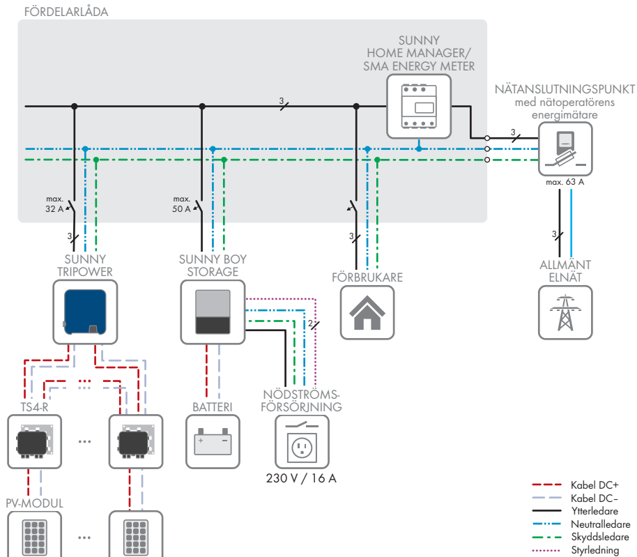
Figur 3: Kopplingsöversikt (exempel)
